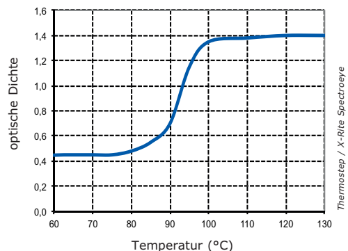
Statische Sensitivität
