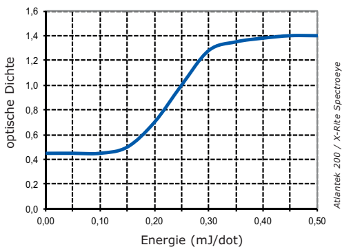
Dynamische Sensitivität
